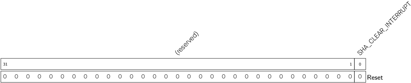
Register 21.6. SHA_INT_CLEAR_REG (0x0024)
