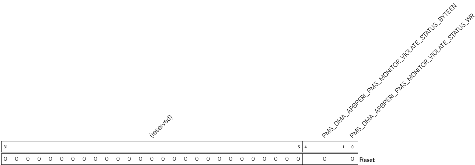
Register 14.63. PMS_DMA_APBPERI_PMS_MONITOR_3_REG (0x008C)
